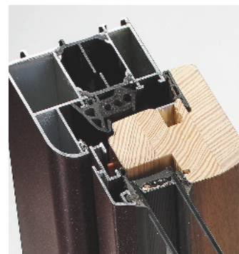
Der Blendrahmen besteht aus thermisch getrennten Aluminiumprofilen, wobei der Flügel in der Kombination Holz-Alu gefertigt ist
