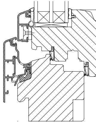
Das Holz-Aluminium-Fenster TimberAlWin 78 ist in geradliniger und profilierter Variante erhältlich
