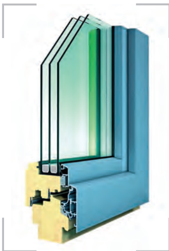
/ Vor allem das „Classicline 88“ von Höhbauer setzt mit 88 mm Bautiefe, Drei-Scheiben-Isolierglas und einem U_w -Wert von 0,80 \text{ W}/(\text{m}^2\text{K}) Maßstäbe.
