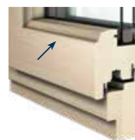
Flügelrahmen „profiliert“
