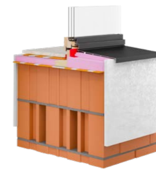
Ziegelmauerwerk verputzt
