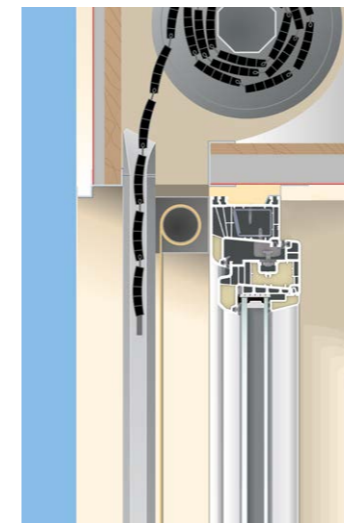
RollaTherm mit integriertem Insektenschutz-Rollo
